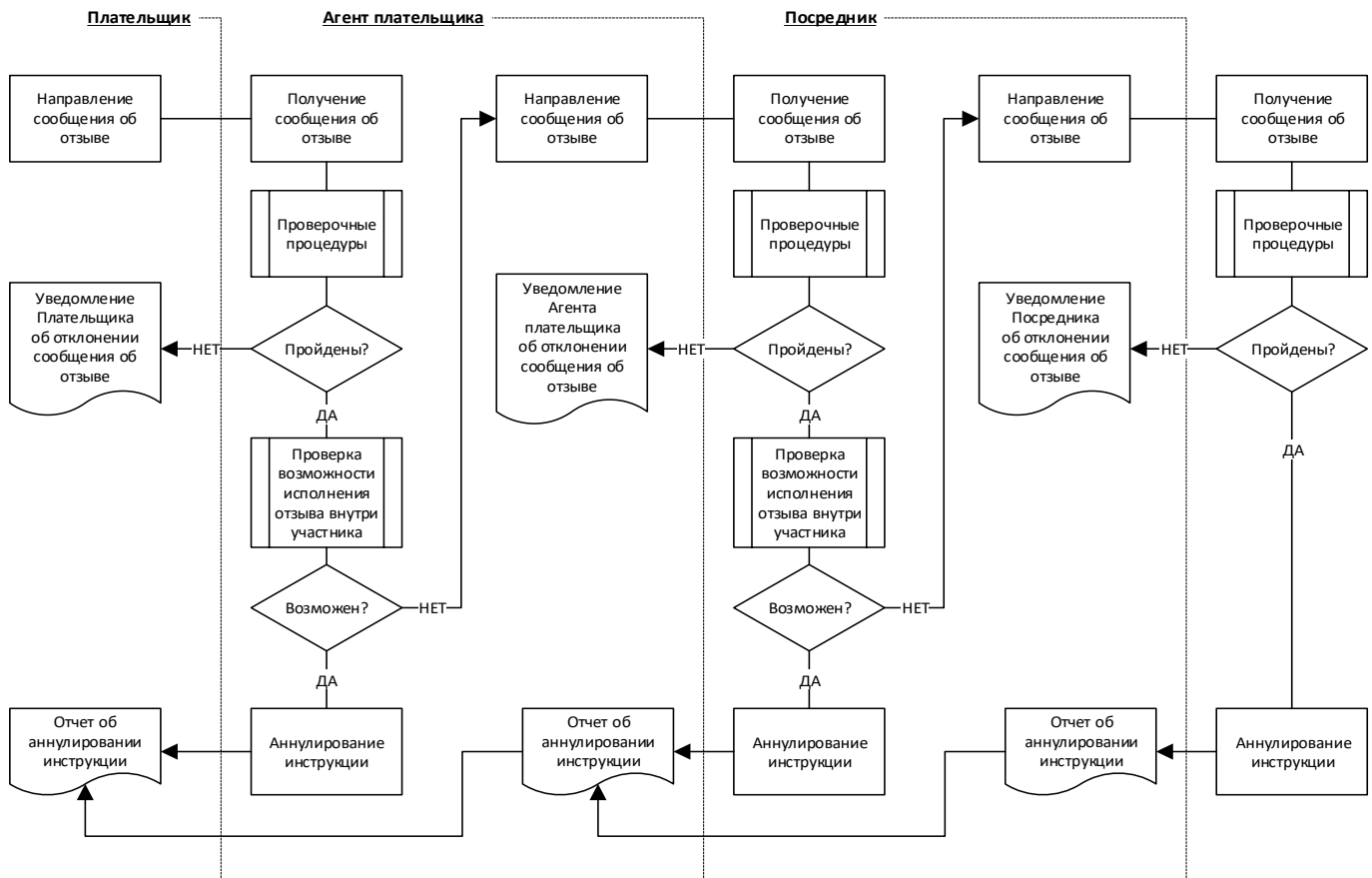
Рисунок 7 – Алгоритм взаимодействия при отзыве инструкции
