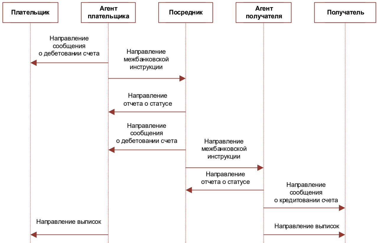
Рисунок 4. Функциональная схема исполнения и подтверждения исполнения инструкции
