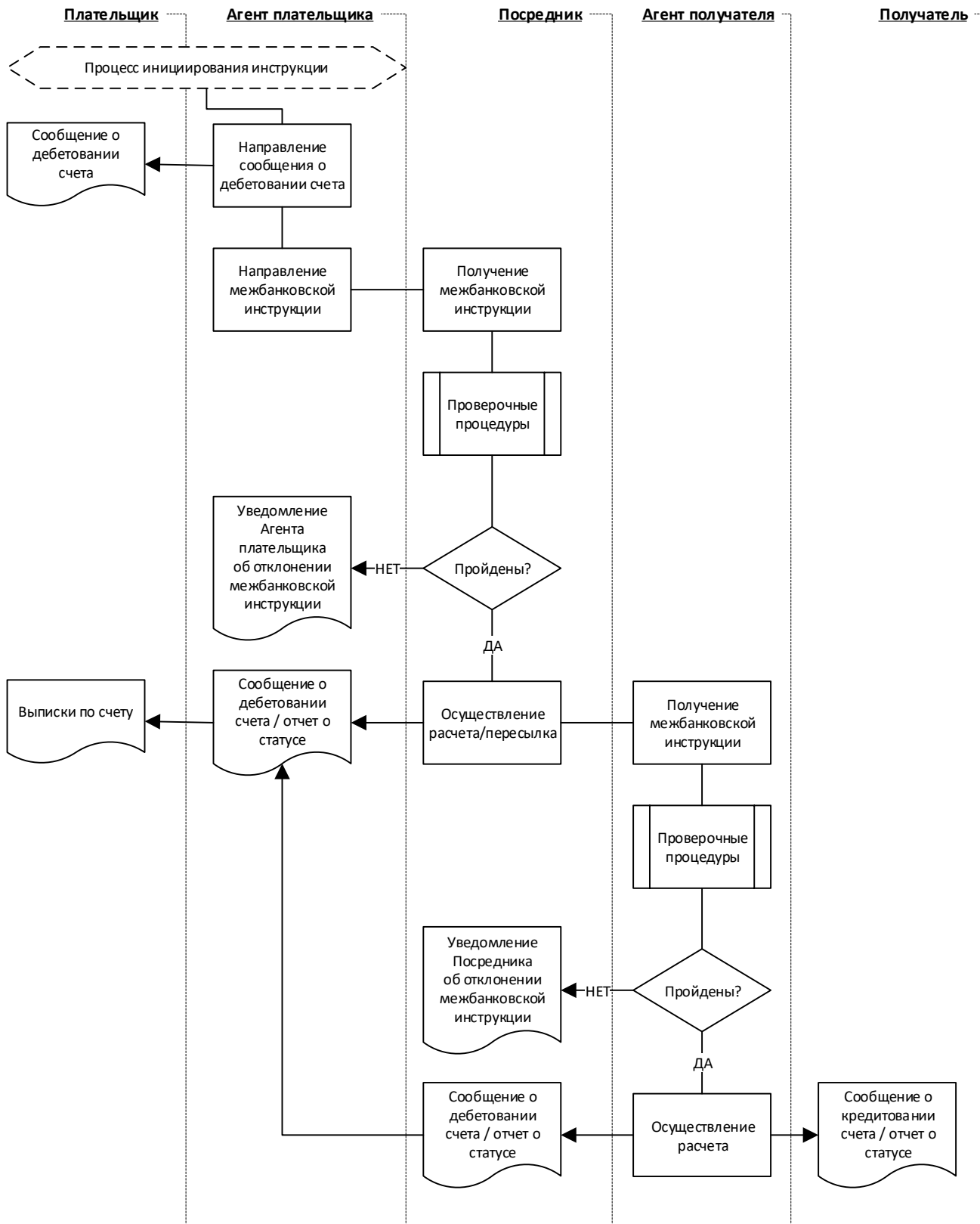
Рисунок 5. Алгоритм взаимодействия при исполнении и подтверждении исполнения инструкции
