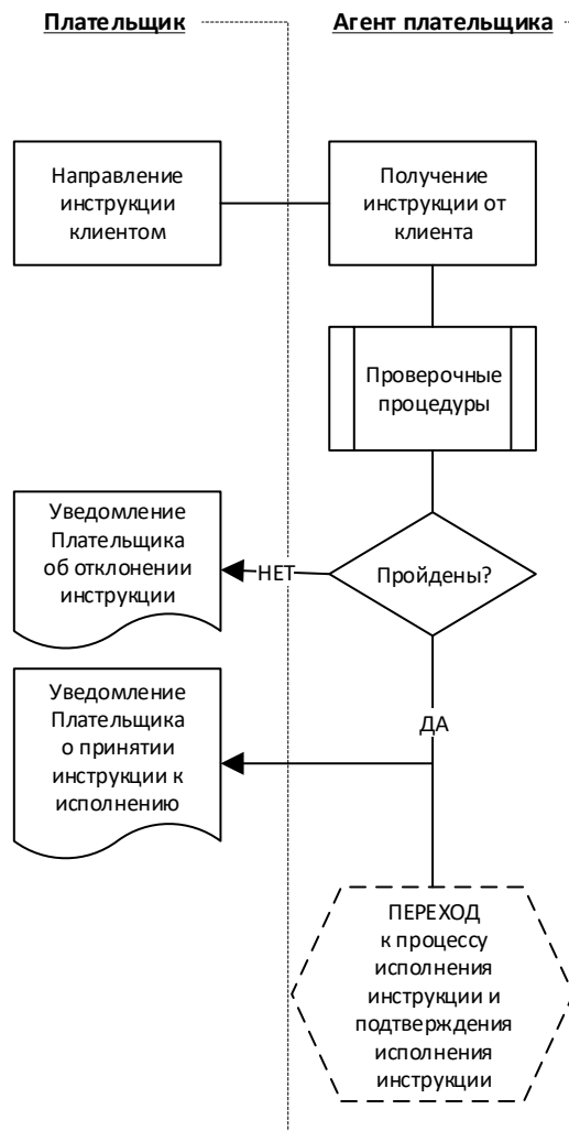
Рисунок 3. Алгоритм взаимодействия при инициировании инструкции
